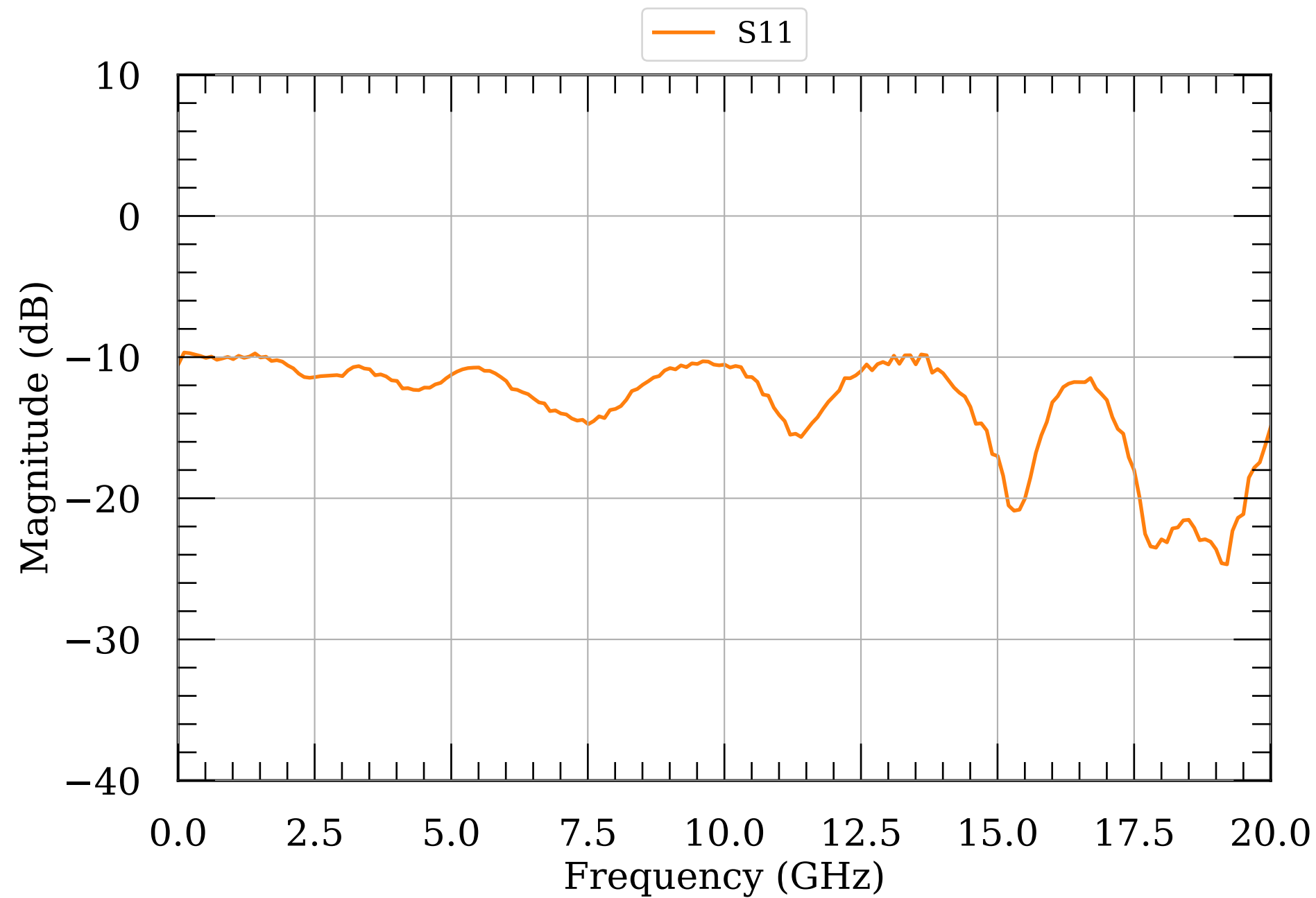
LNA S-params module008
